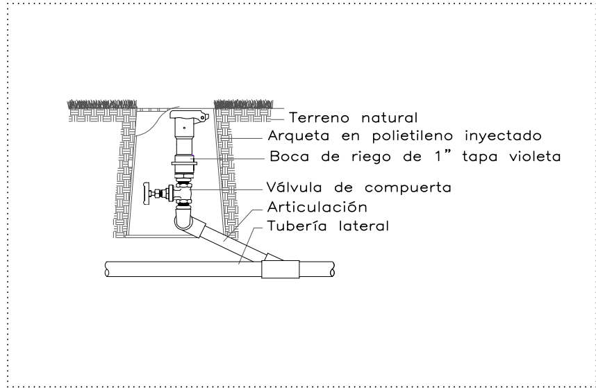
DETALLE 01 _ BOCAL DE RIEGO ENLACE RÁPIDO (SIN ESCALA)
