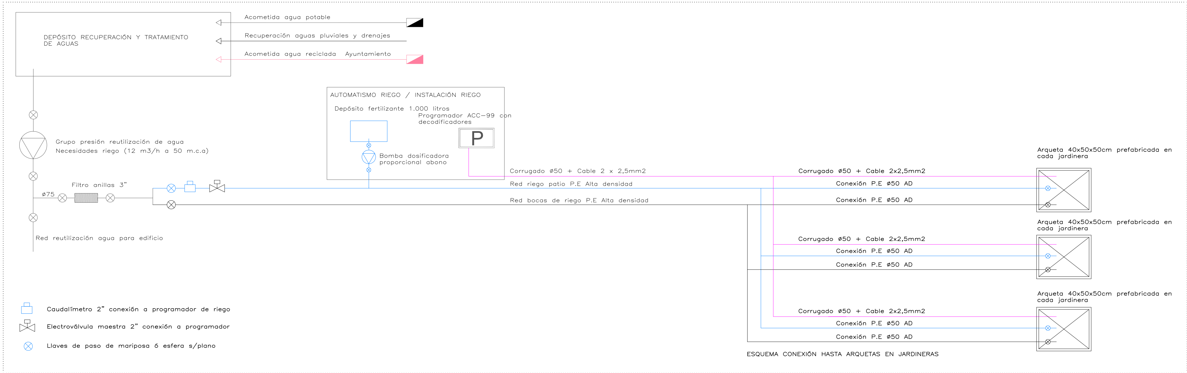
DETALLE 09 _ ESQUEMA CONEXIÓN EN SALA TÉCNICA
