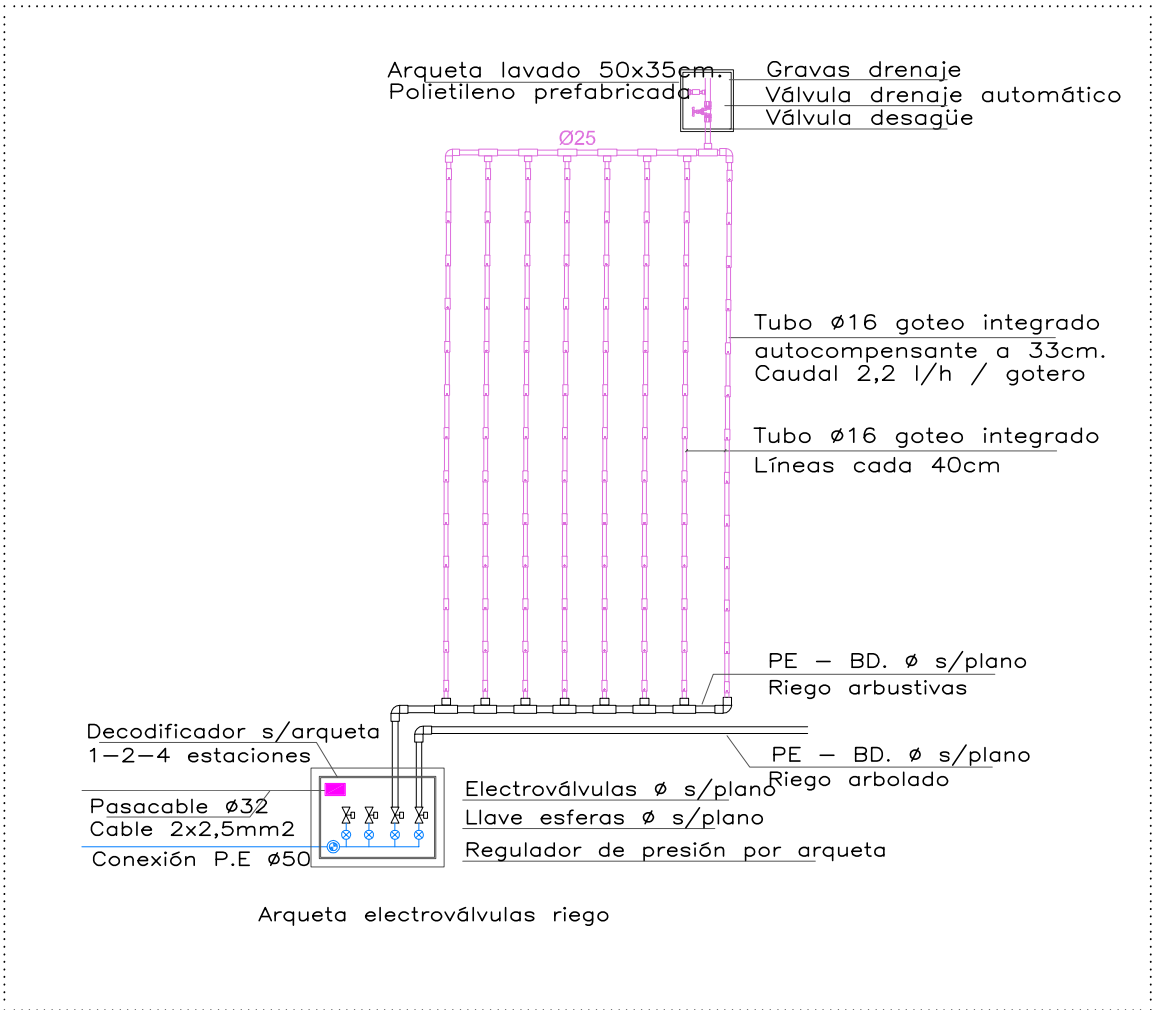
DETALLE 06 _ ESQUEMA RIEGO GOTEO ARBUSTIVAS (SIN ESCALA)
