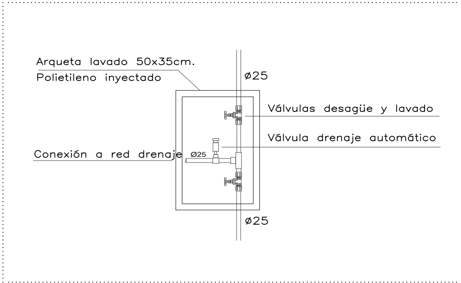
DETALLE 03 _ ARQUETA DRENAJE GOTEO (SIN ESCALA)
