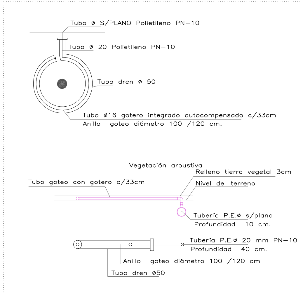
DETALLE 05 _ RIEGO ARBOLADO Y ARBUSTIVAS (SIN ESCALA)
