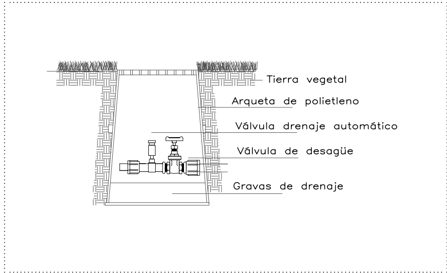
DETALLE 04 _ ARQUETA DRENAJE FASES DE GOTEO (SIN ESCALA)
