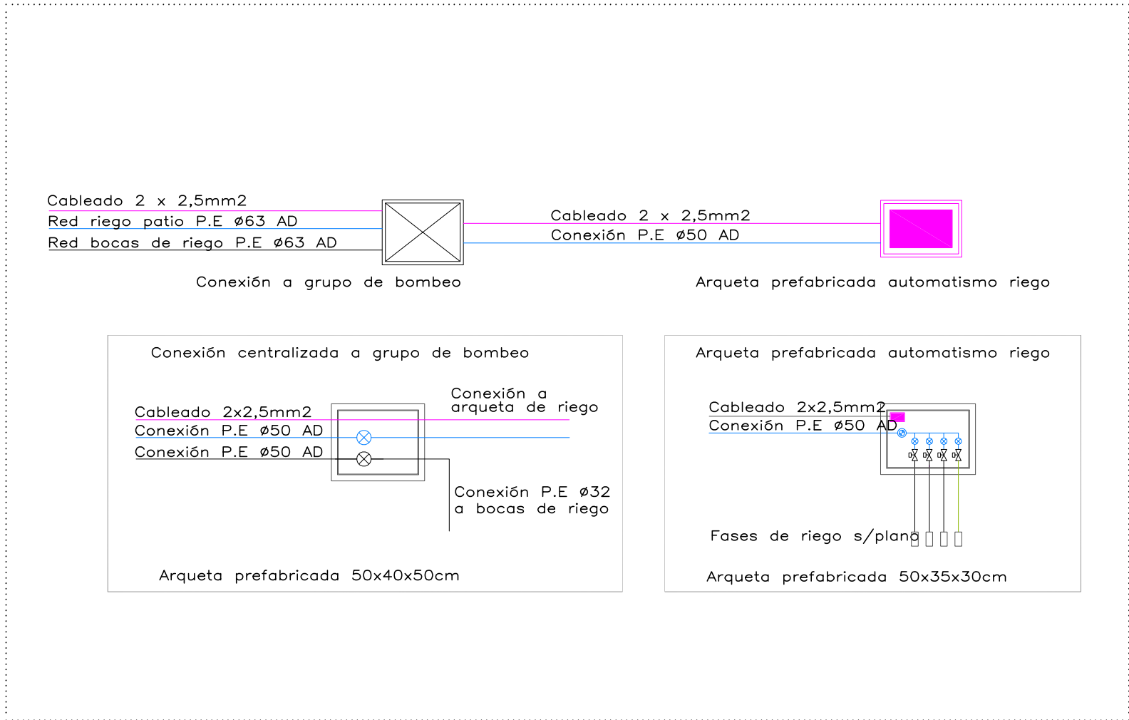
DETALLE 07 _ ACOMETIDA DE AGUA
