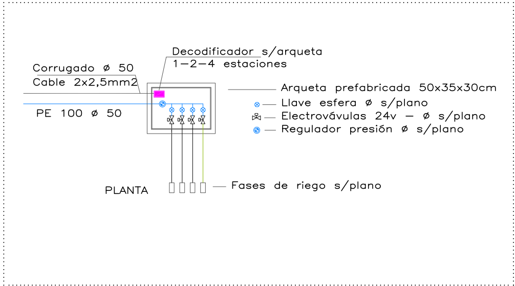
DETALLE 02 _ ARQUETAS ELECTROVÁLVULAS (SIN ESCALA)
